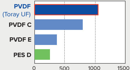
中空糸膜の機械的強度 (g/Fiber)
