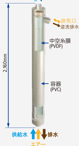
加圧型UF膜モジュール (HFUG/HFU)
